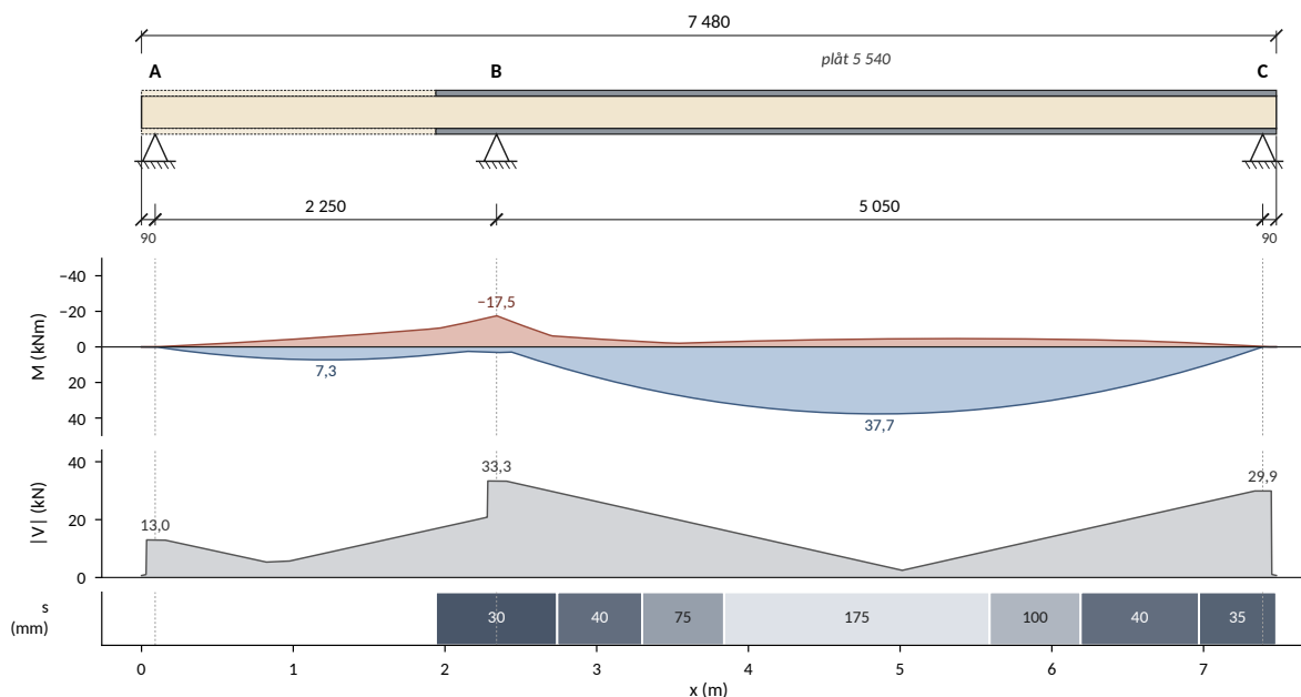
Figur 5: Dalbalk 4. Stöd, plåtbitar, omhüllande moment (ritat på dragen sida) och tvärkraft i brottgränstillstånd för samtliga modeller och lastfall, med och utan limverkan, samt skruvdelning s längs plåten (mm).
