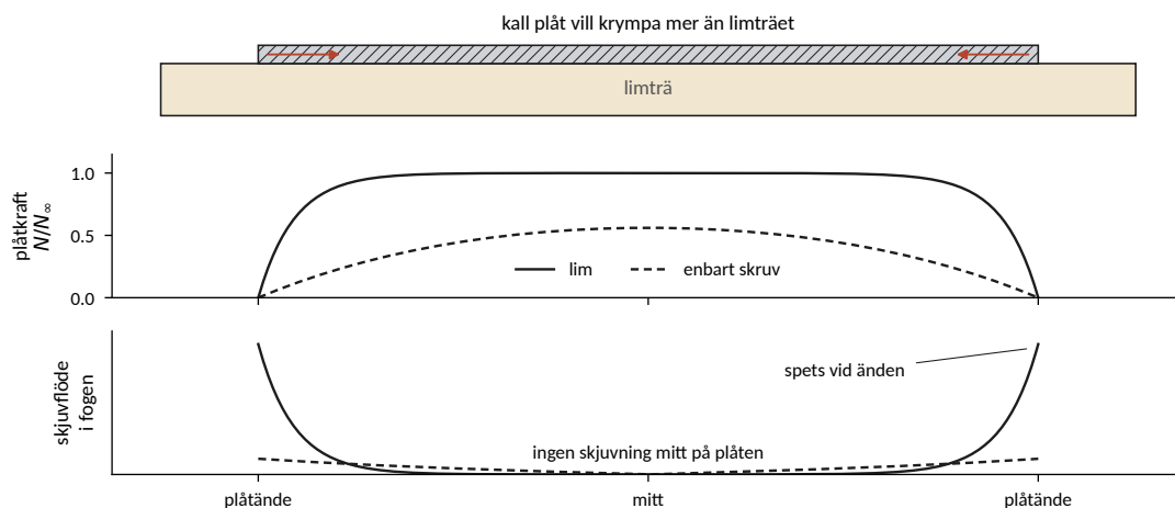
Figur 1: Plåtkraft och skjuvflöde i fogen längs en 4 m lång plåt när plåtarna kyls lika mycket.
